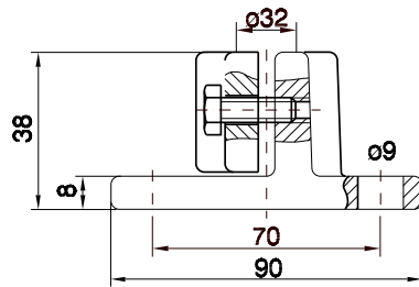
Anschlagflansch 32
