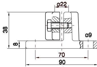
Anschlagflansch 22
