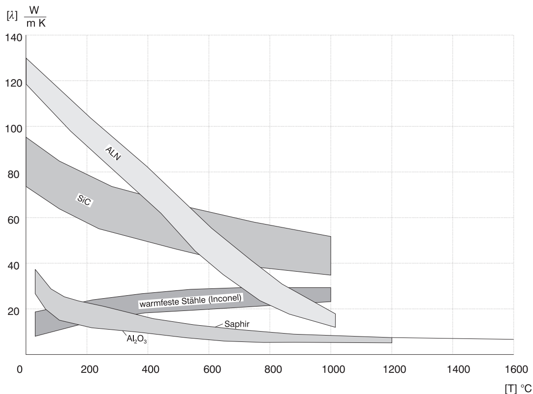
Wärmeleitfähigkeit verschiedener Stoffe
